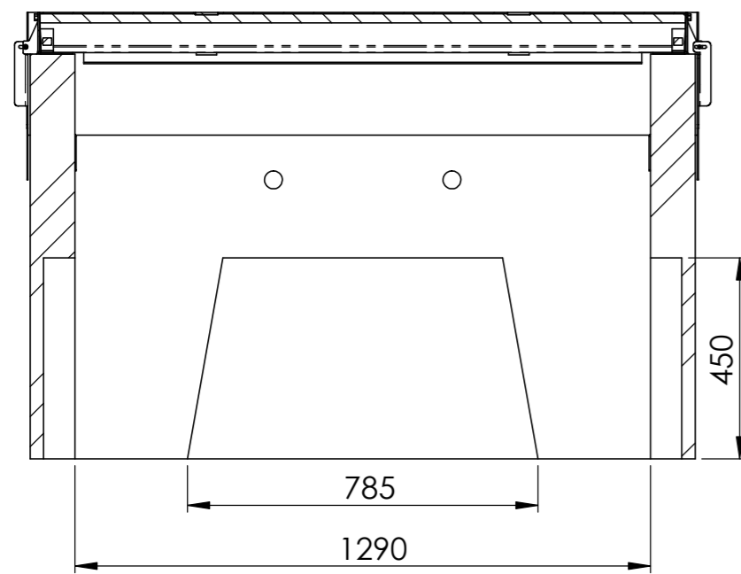
SCHNITT B-B MABSTAB 1 : 15
