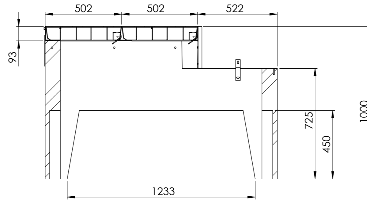
SCHNITT A-A MABSTAB 1 : 15
